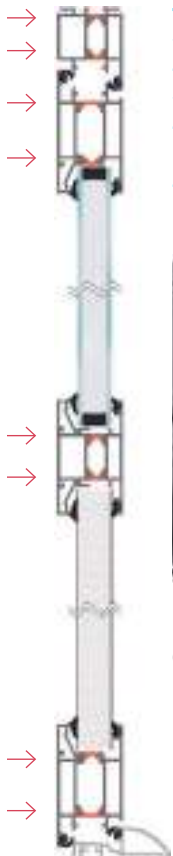
Profilés à double feuillure et rupture de pont thermique
